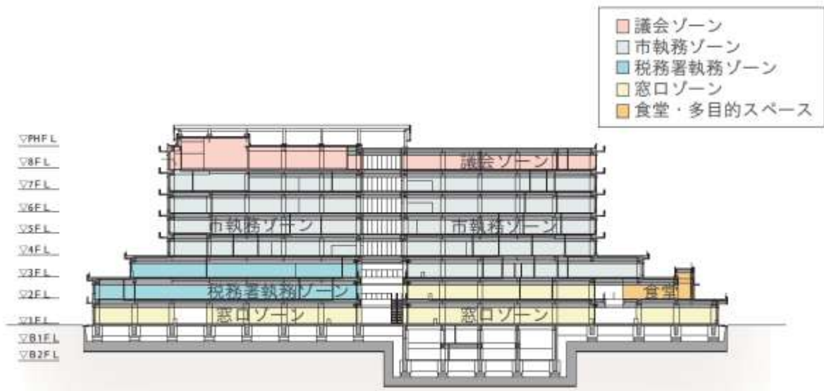
階構成図
