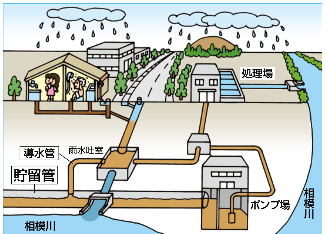
△図2 合流式の改善工事後の仕組み
