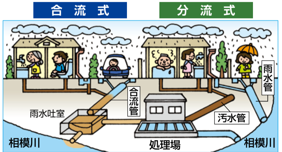
△図1 合流式と分流式の仕組み
