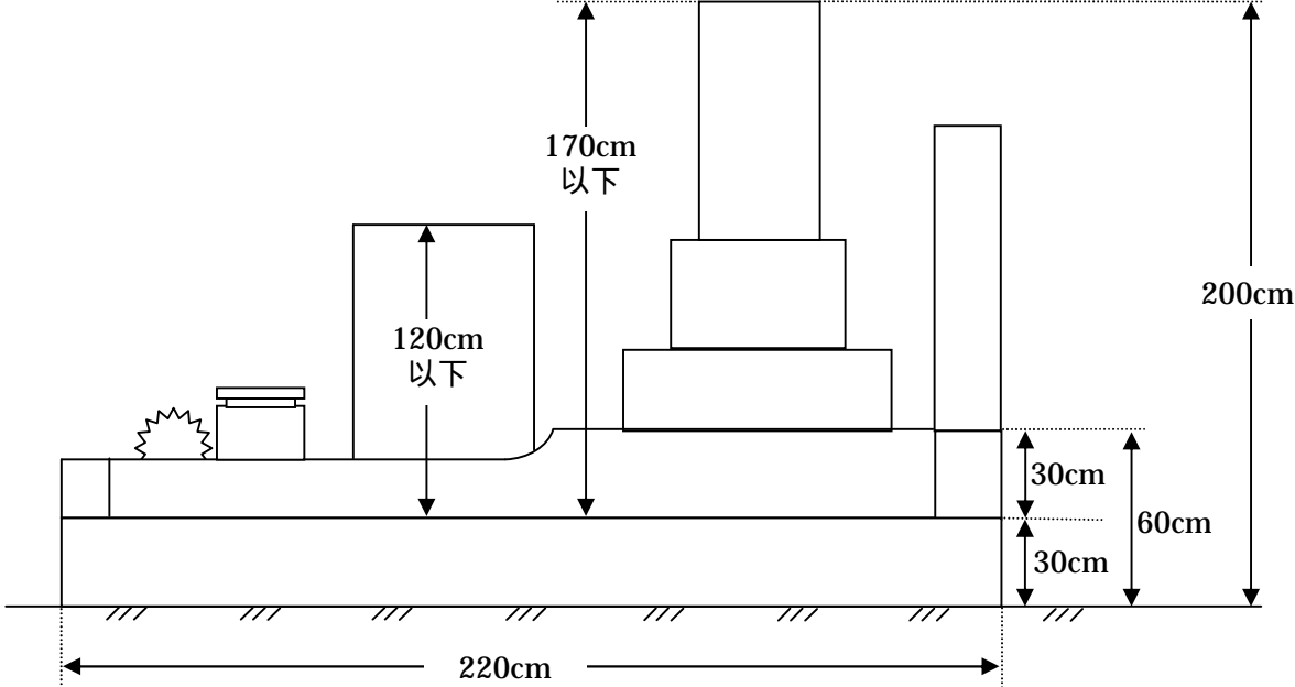
側面図
