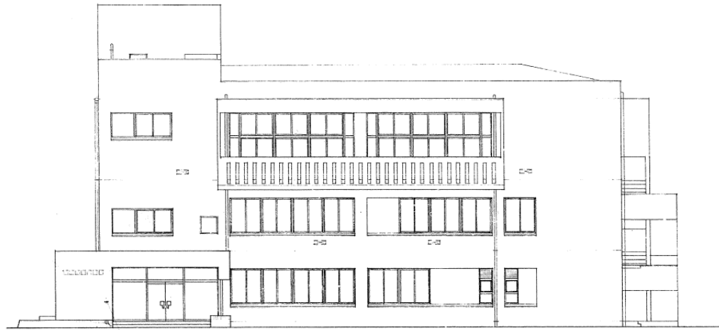
東側立面図
