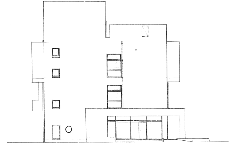
南側立面図
