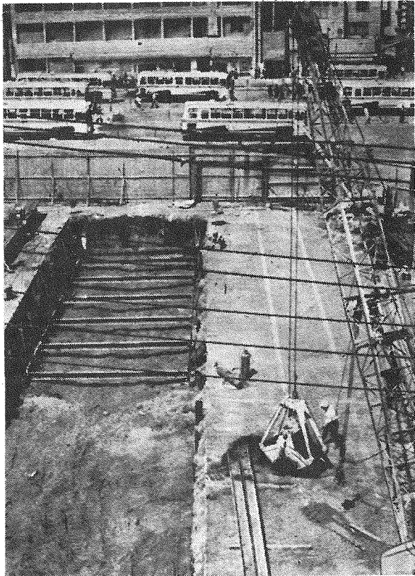
駅前広場改修工事・ご存知の駅前広場の下に地下道をつくらうという工事。44年度いっぱい主要工事ができ上るといふから、来年の4月以降は利用できそう。
