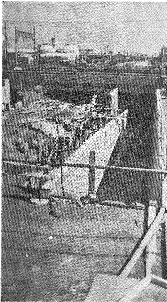
江陽中学校プール・7月20日完成の予定で、いまちょうど半ほどの工を進行中。15坪×25坪のプールで水しぶきをあげようと、江陽の若者たちは首を長くして待つている。
