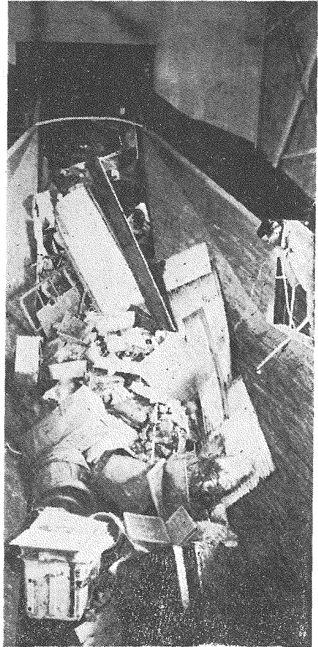
収集車で運びこまれたごみは、はじめにこの投入口にはいる。投入されるときはシャワーで万全
