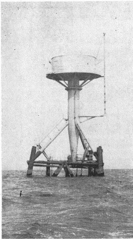
全国初の観測器を備えた波浪等観測塔…水面上20M。建設費7300万円、60Mの風速に耐える。漁船の接近と泳いでいく人が観測をさまたげるのが悩み。
