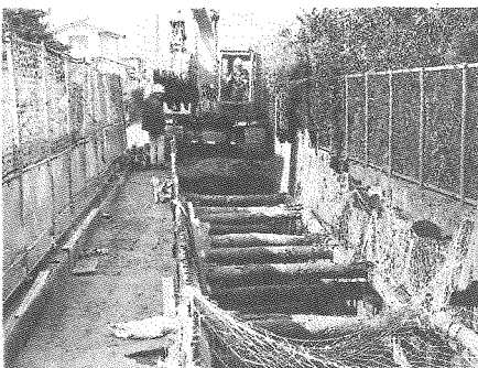
神明中学校前の公共下水道工事
