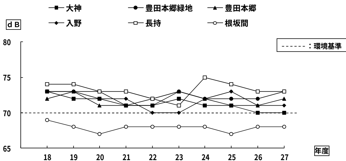
図3-7 新幹線騒音測定結果経年変化
