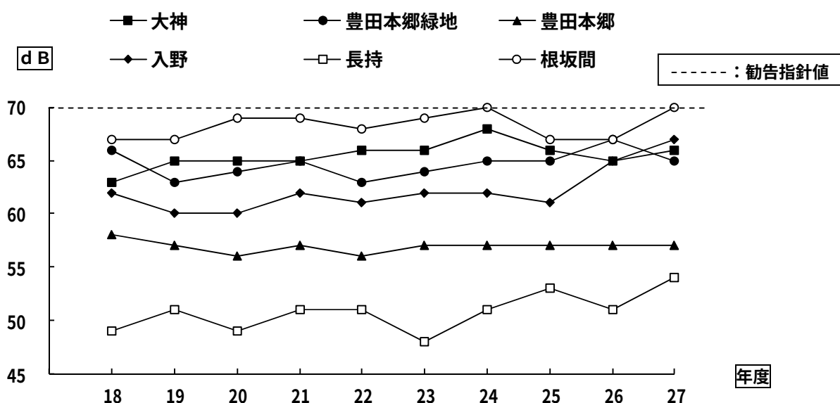
図3-8 新幹線振動測定結果経年変化
