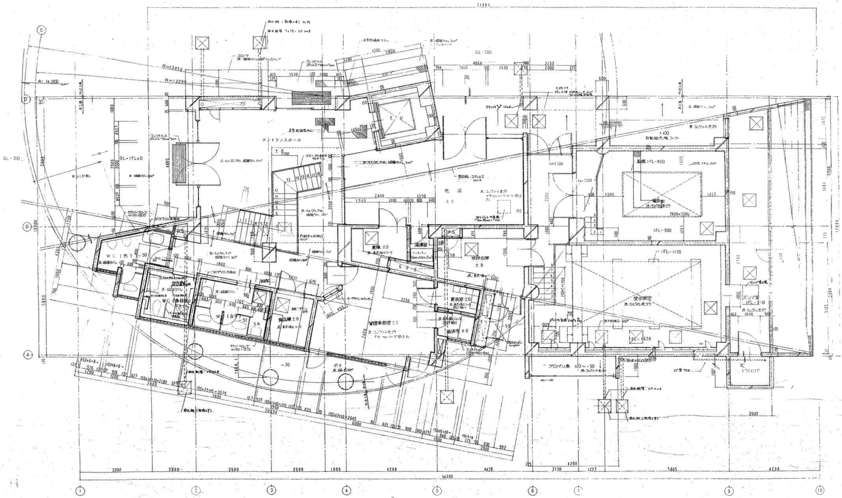
1階平面詳細図
