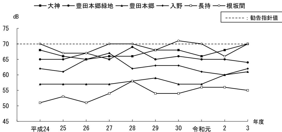
図3-8 新幹線振動測定結果経年変化
