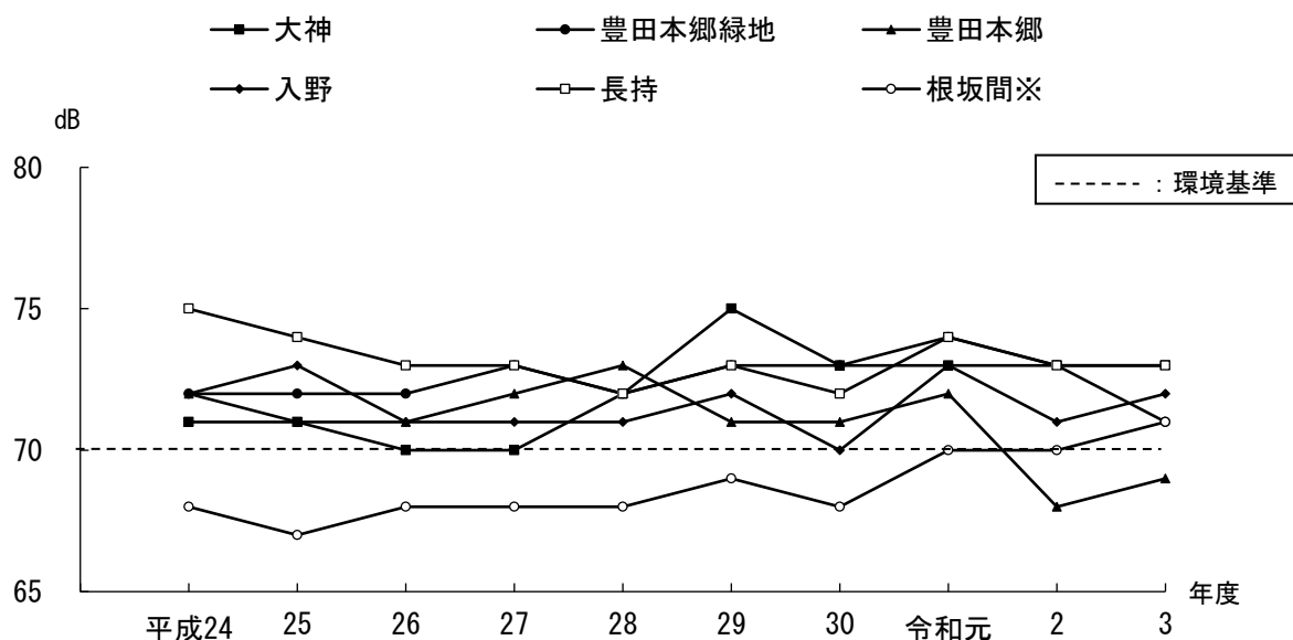
図3-7 新幹線騒音測定結果経年変化
