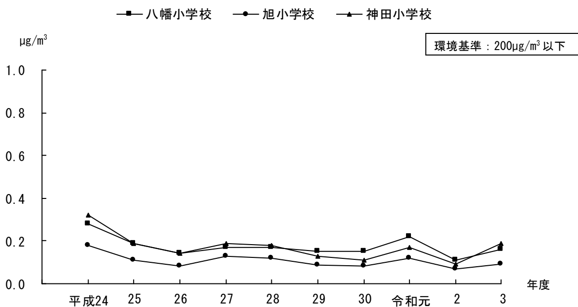
図 1-12 テトラクロロエチレンの経年変化（1年平均値）
