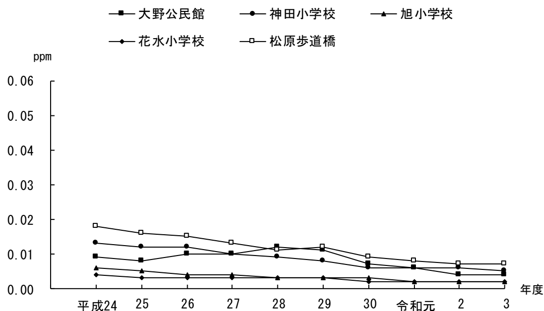
図 1 - 3 一酸化窒素の経年変化 (年平均値)
