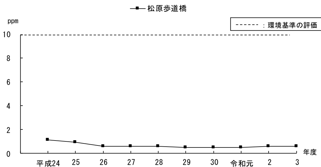
図1－5 一酸化炭素の経年変化（日平均値の2%除外値）
