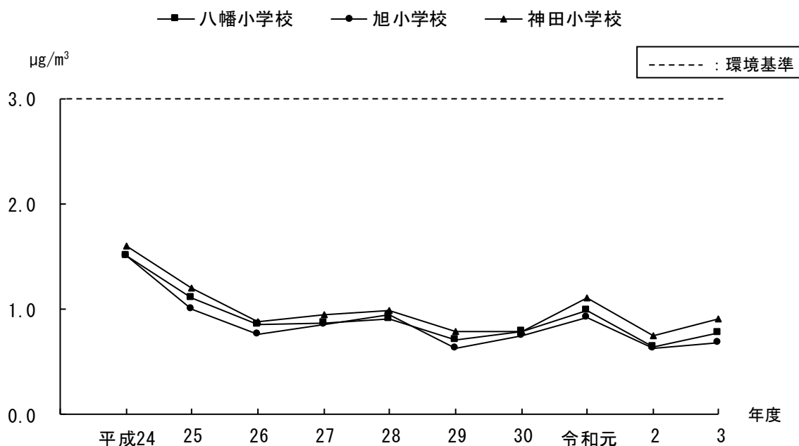
図1-10 ベンゼンの経年変化（1年平均値）
