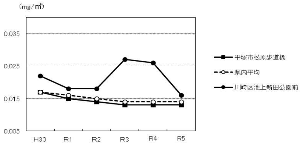
浮遊粒子状物質濃度の経年推移 (自動車排出ガス測定局(注2)における年平均値)
