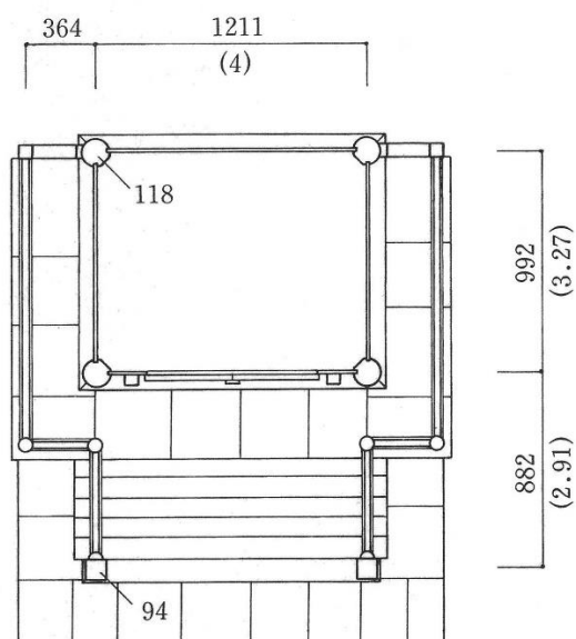
図1 実測図
