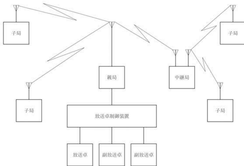
回線構成図
