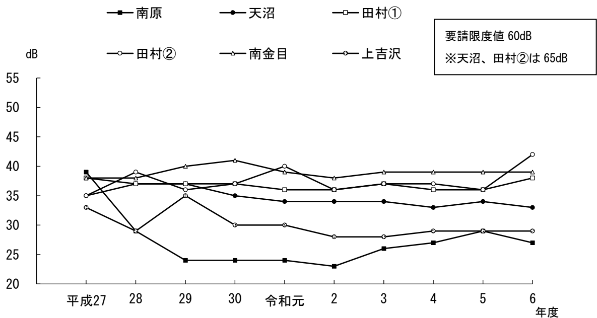
図3-5 自動車振動測定結果経年変化（夜間）
