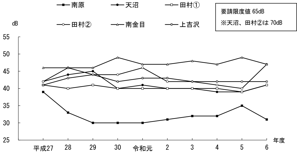
図3-4 自動車振動測定結果経年変化（昼間）
