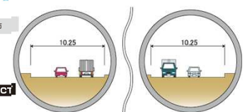
トンネル部 (A-A')
