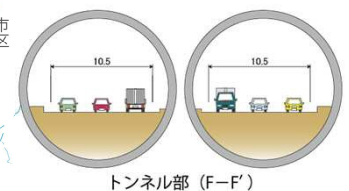
トンネル部 (F-F')
