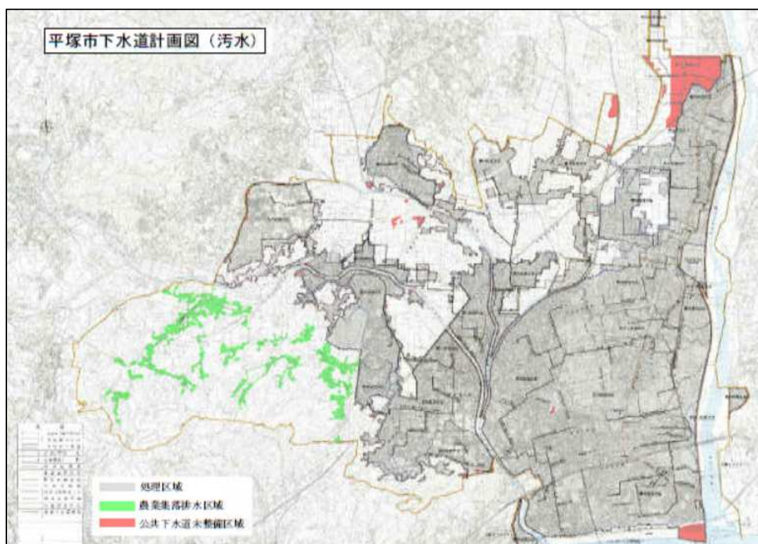
図 3-2 平塚市下水道計画図（污水）
