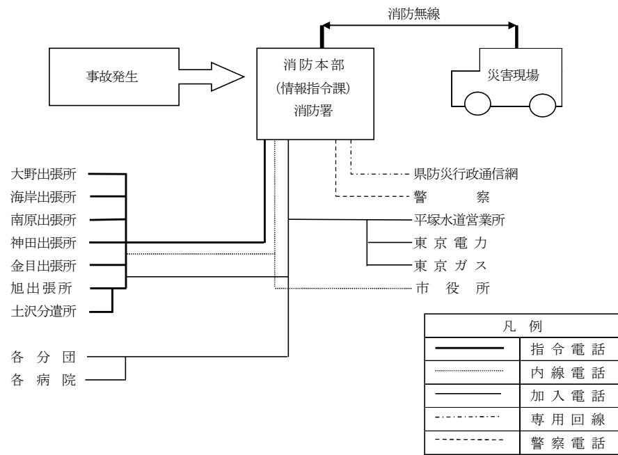
消防出場系統図
