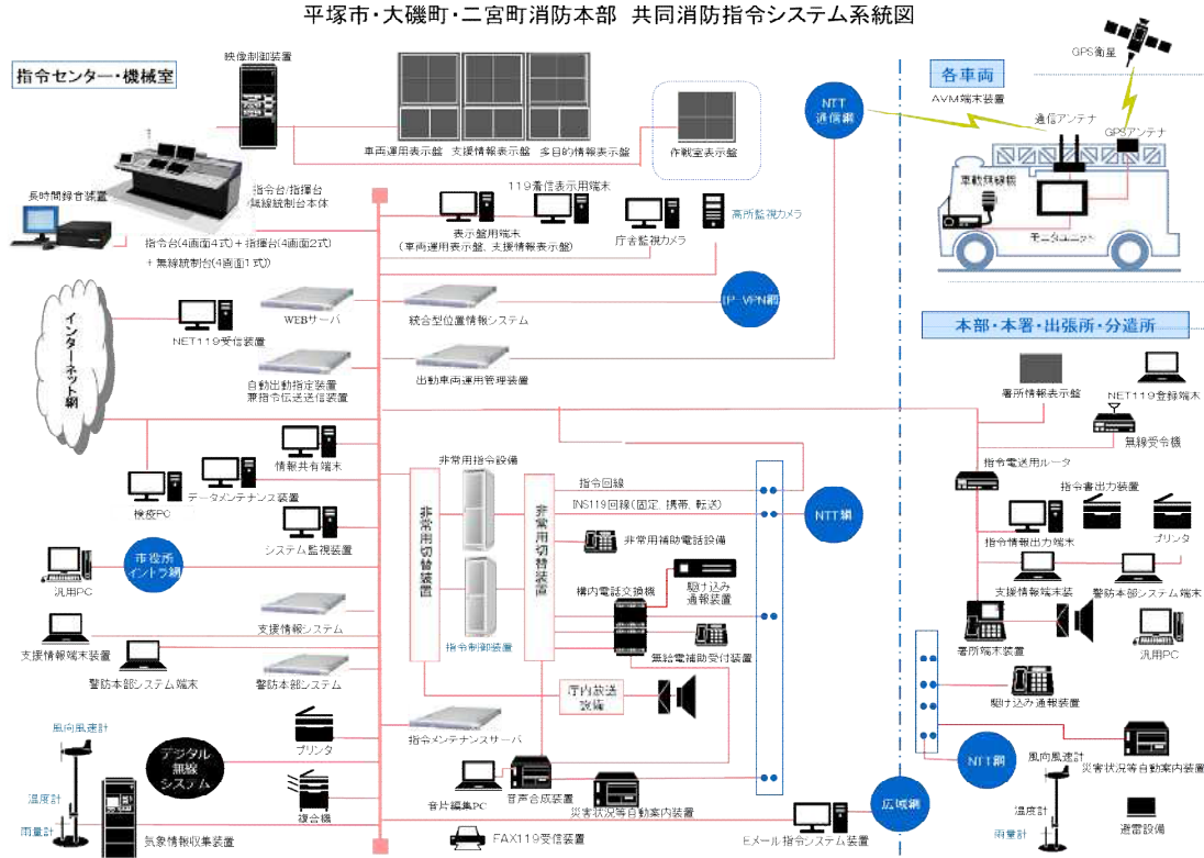
平塚市・大磯町・二宮町消防本部 共同消防指令システム系統図
